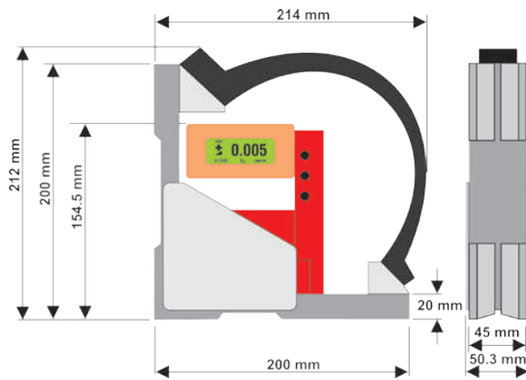
BlueLEVEL BASIC with horizontal base and wireless transmission mit horizontaler Messbasis und mit Datenübertragung per Funk
