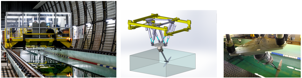
FIGURE 1 – Vue du dispositif expérimental.
