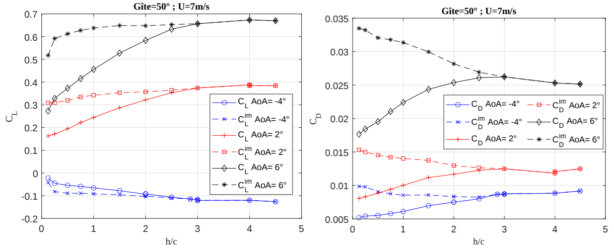
FIGURE 8 – C_L et C_d vs \frac{h}{c} pour plusieurs AoA à Gîte = 50^\circ et U = 7 \text{ m.s}^{-1} ; trait plein : C_i définis par rapport à la surface totale de l'aile; trait pointillé : C_i^{im} définis par rapport à la surface immergée de l'aile.
