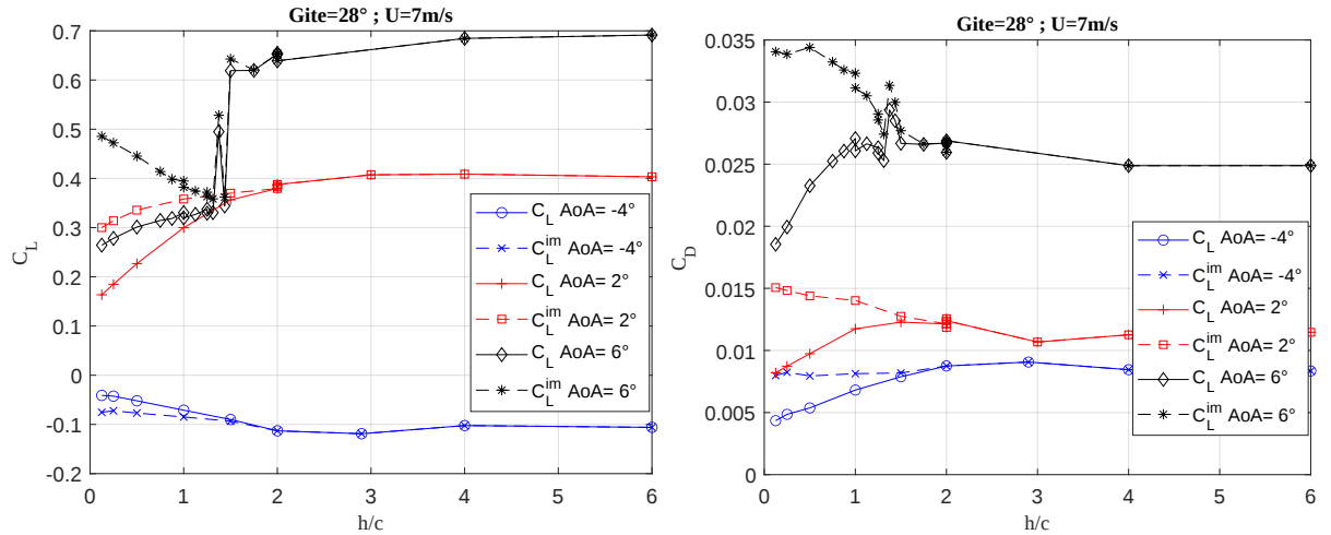
FIGURE 9 – C_L et C_d vs \frac{h}{c} pour plusieurs AoA à Gîte = 28^\circ et U = 7 \text{ m.s}^{-1} ; trait plein : C_i définis par rapport à la surface totale de l'aile; trait pointillé : C_i^{im} définis par rapport à la surface immergée de l'aile.
