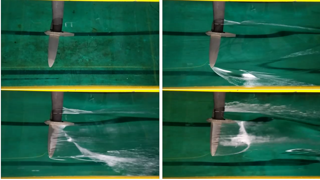
FIGURE 10 – Cas de ventilation sur l’aile elliptique ( G\acute{a}te = 28^\circ ; \frac{h}{c} = 0.375 ; AoA = 6^\circ : U = 7m.s^{-1} .
